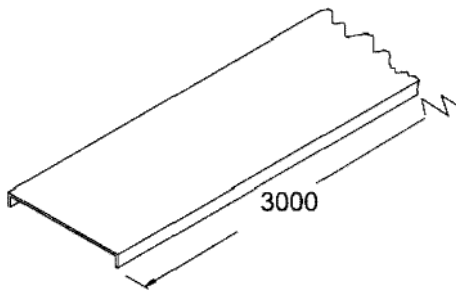
Tampa de Encaixe para Perfilado Duplo 76x3000mm
