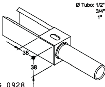
Saída Final para Eletroduto
