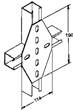
Junção Plana "X" Reforçada
