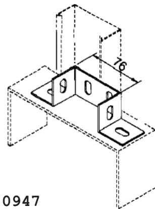
Base Dupla para Ligação em Painel
