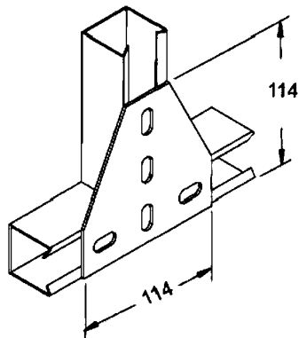
Junção Plana "T" Reforçada
