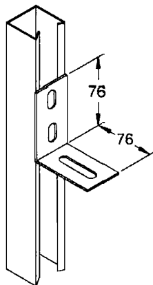
Cantoneira com 2 Furos e 1 Rasgo
