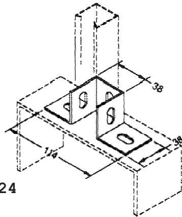
Base para Ligação em Painel
