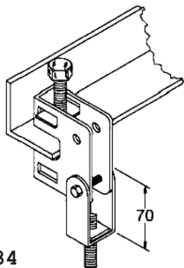
Balancim para Grampo "C"
