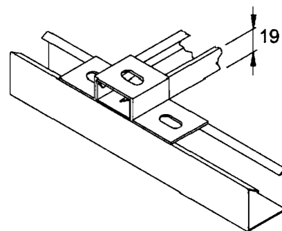
Cantoneira "ZZ" Meia
