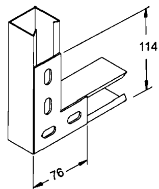
Junção Plana "L"
