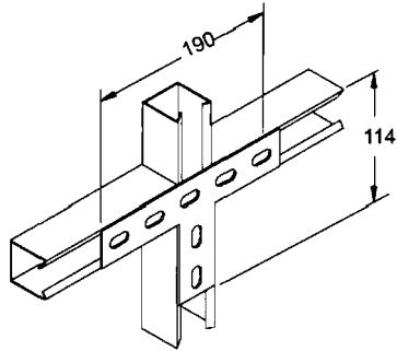
Junção Plana "T"
