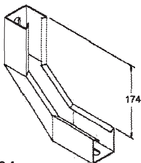
Curva Vertical Interna 90° para Perfilado 38x38
