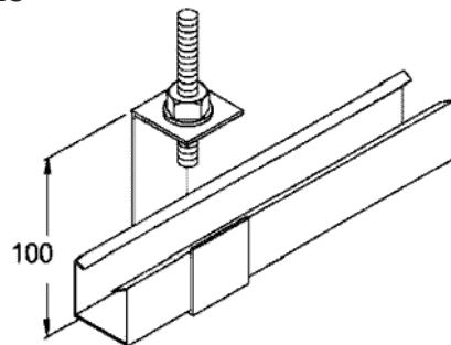
Gancho Curto para Perfilado
