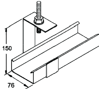
Gancho Longo para Perfilado 38x76
