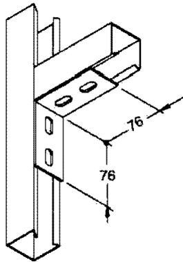
Cantoneira com 4 Furos Simples
