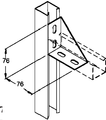
Cantoneira com 4 Furos Reforçada
