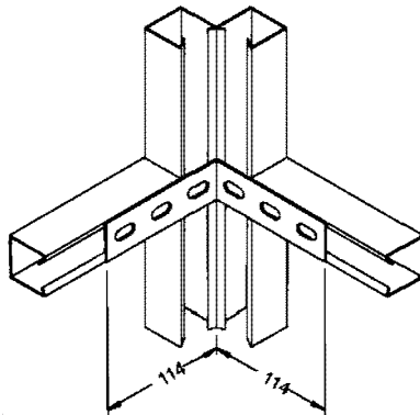
Cantoneira com 6 Furos Simples
