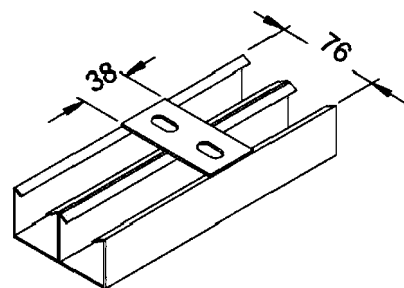
Tala Simples com 2 Furos
