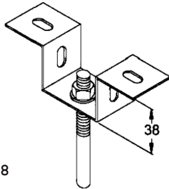
Cantoneira "ZZ" para Vergalão
