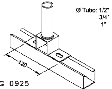
Saída Superior para Eletroduto
