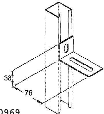
Cantoneira com 1 Furo e 1 Rasgo
