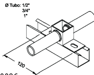
Saída Lateral Dupla para Eletroduto
