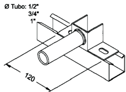
Saída Lateral Simples para Eletroduto
