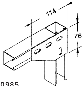
Junção Plana "L" Reforçada
