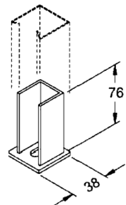
Base Interna com 1 Furo
