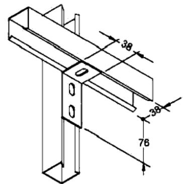
Cantoneira com 3 Furos Simples
