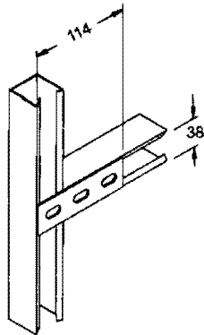
Tala Simples com 3 Furos
