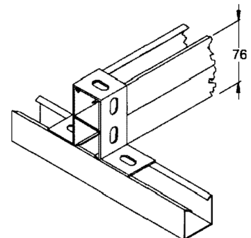
Cantoneira "ZZ" Dupla Vertical
